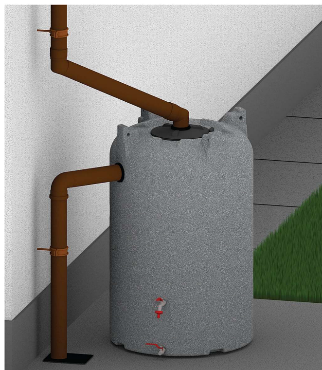
Telepítési példa az AQUATOWER 0,5 tartály alapján
